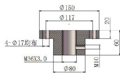
法兰端FL Flange end FL
