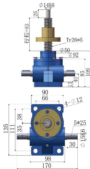
E 螺母在上 E Upright rotating screw
